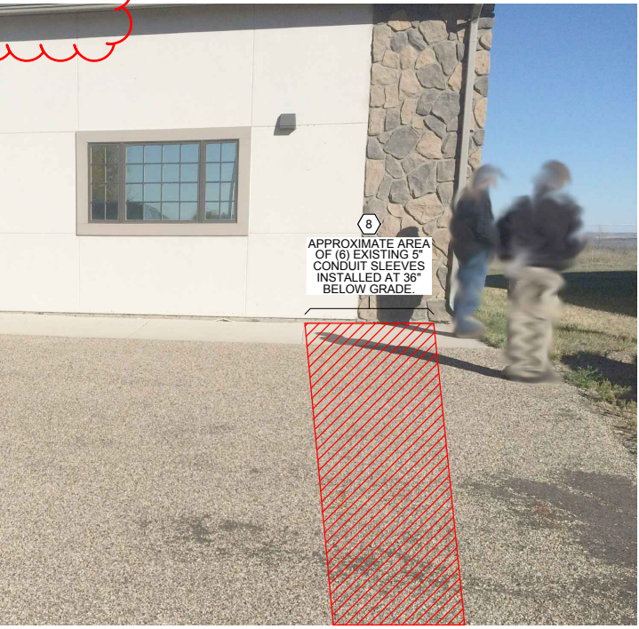
2 CONDUIT LOCATION PHOTO
